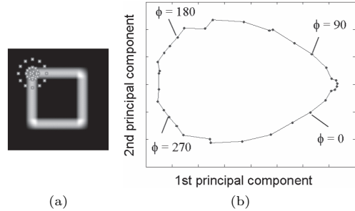
図 3 (a) テスト画像とサンプリング点配置, (b) 特徴量空間
